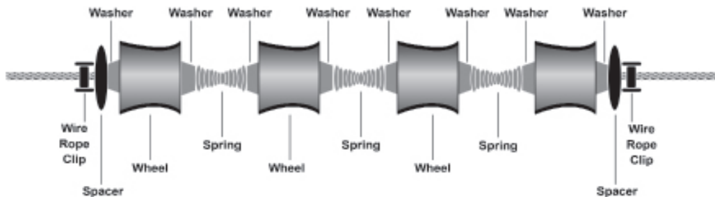
PN 2002 - Pipe Sling
